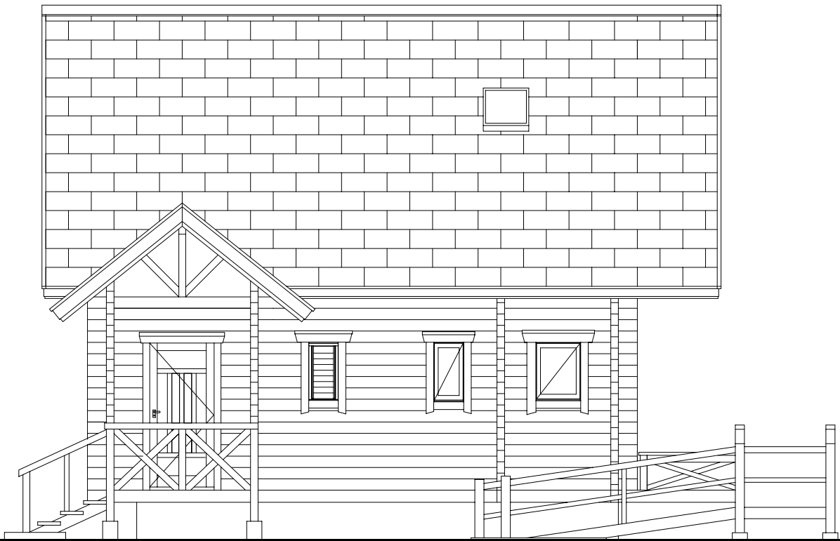
西立面图
